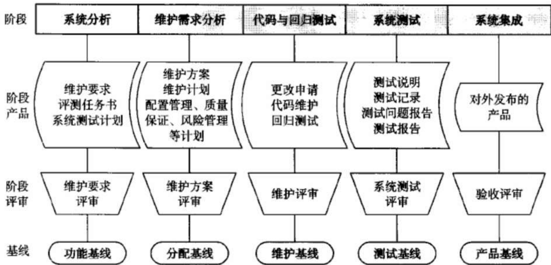
图2 软件维护过程
