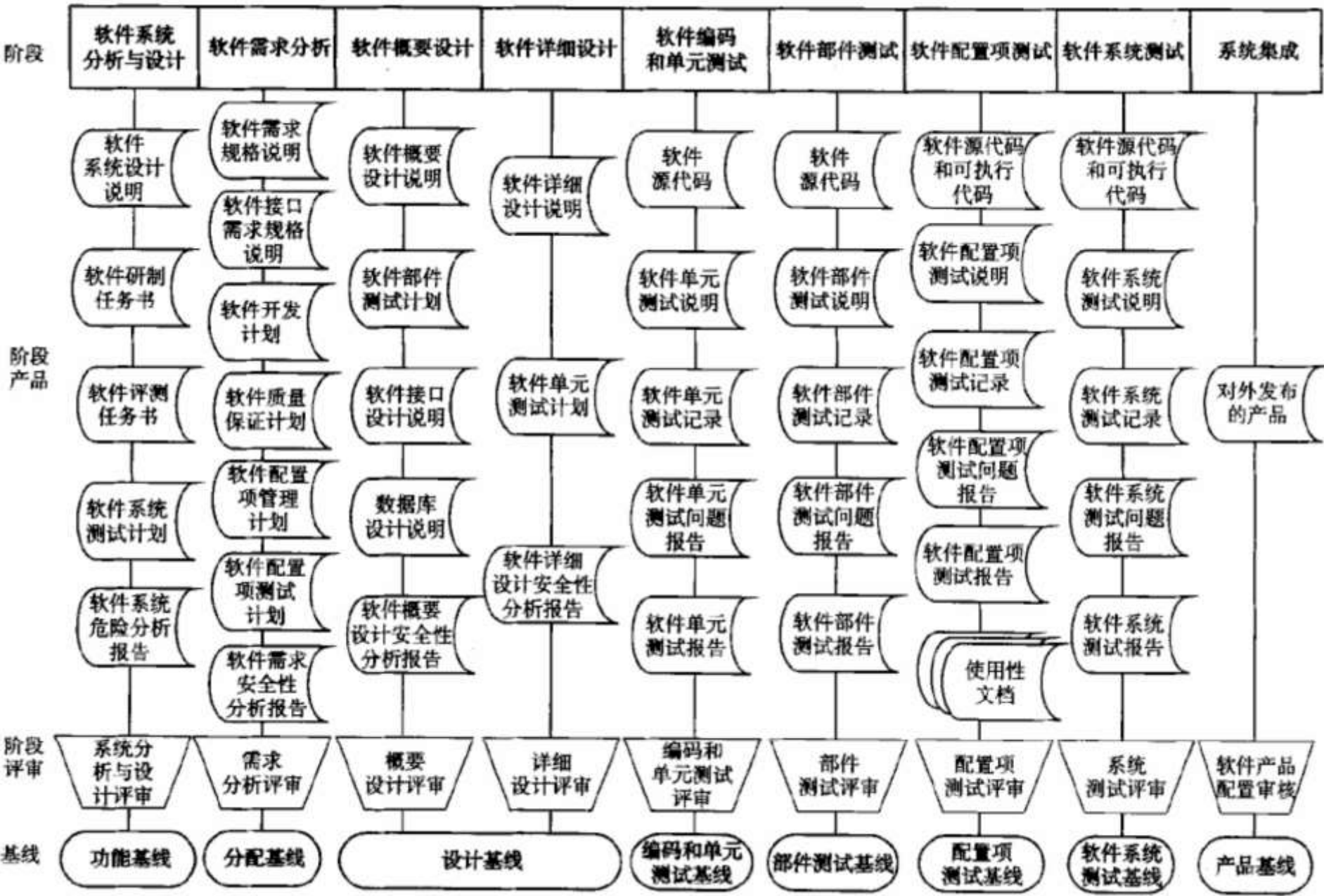
图1 软件开发过程
